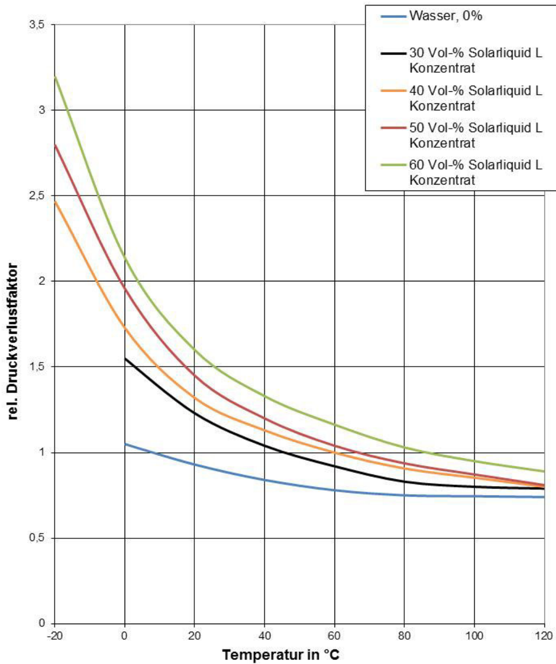
rel. Druckverlustfaktor von Solarliquid L Konzentrat/ Wassermischungen in Abhängigkeit von Temperatur und Konzentration
